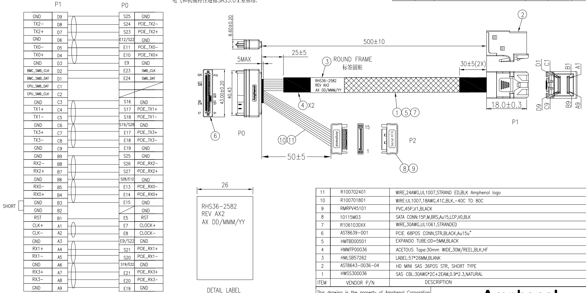
WIRING TABLE
